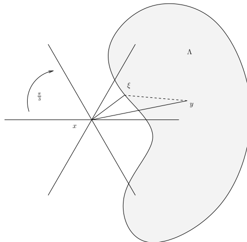
Fig. 8.1. The geometric argument in Lemma 8.17.
